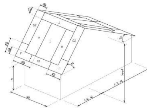
4. Ongelijkzijdig zadeldak
