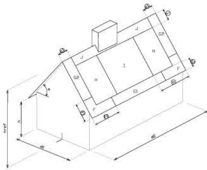
1. Zadeldak
