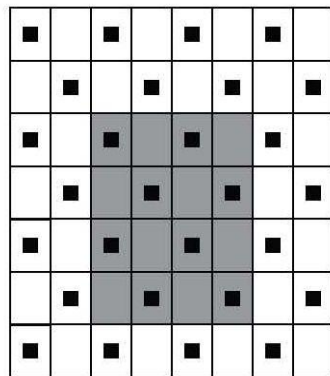
Dambordgewijs verankeren van dakpannen
