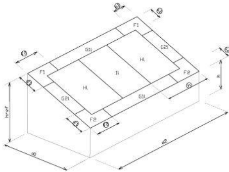
9. Lessenaarsdak
