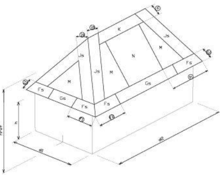
3. Vierzijdig zadeldak
