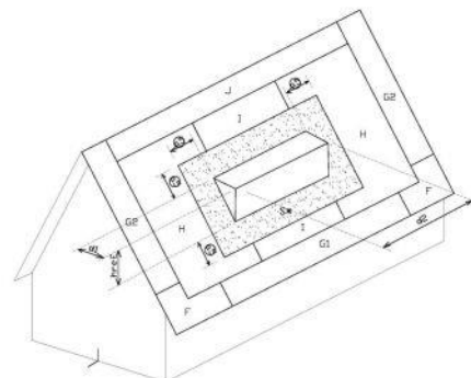
14. Dakkapel
