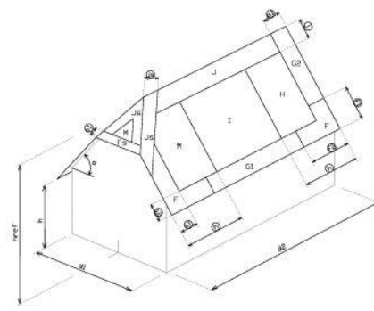
2. Zadeldak met wolfseind
