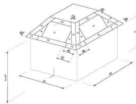
12. Afgeknotte pyramidak
