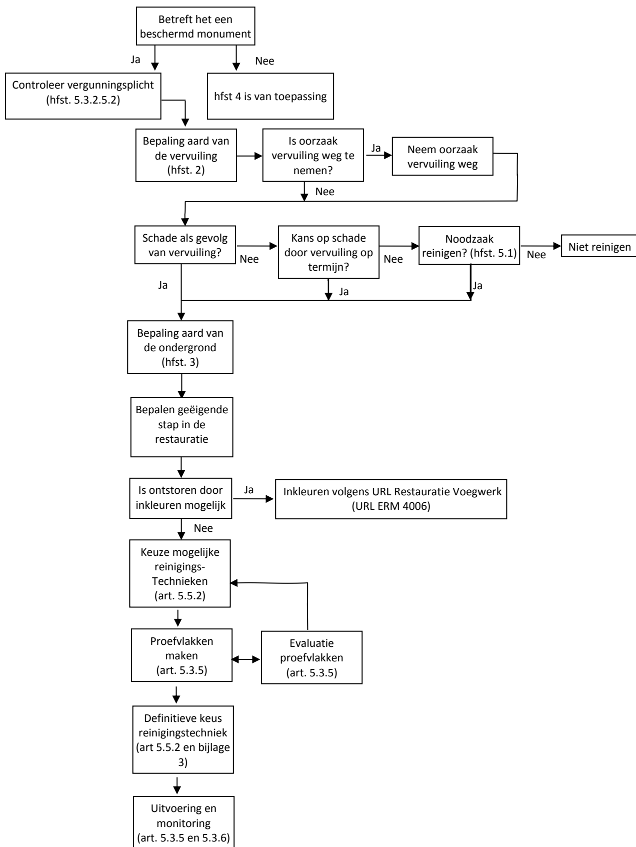
Figuur 5.1 Stappenplan gevelreiniging restauratie
